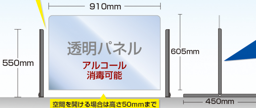
正面図
